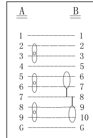
WIRING TABLE:
